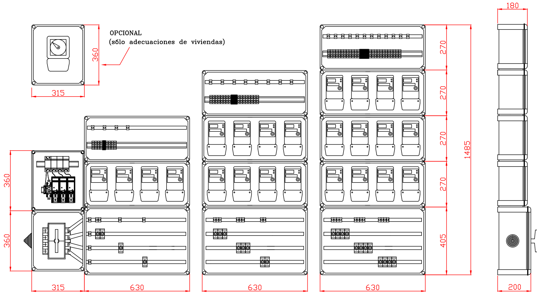
CENTRALIZACION MODULAR MONOFASICA BIDIRECCIONAL ERZ CMM2008
