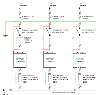
ESQUEMA ELÉCTRICO
