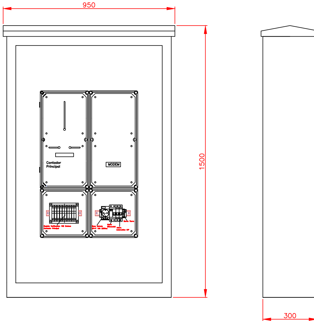
PNZ-ARMARIO METALICO+MODULO AT FECSA-ENDESA (AT<36kV)
