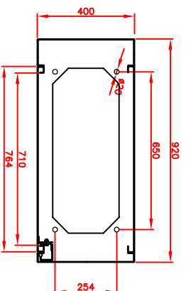
SECCION A-A'
