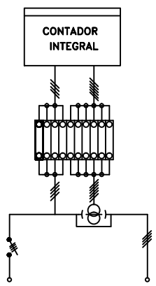
ESQUEMA ELECTRICO
